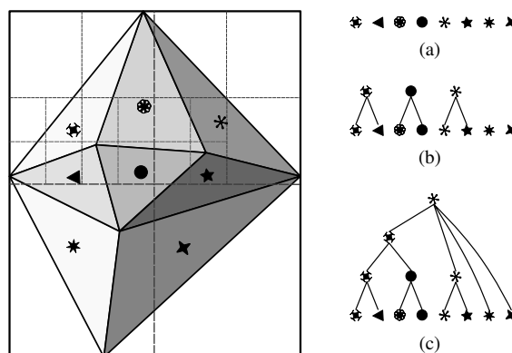
Figure 4: Construction de la hiérarchie : à gauche, l'objet plongé dans un octree avec une face (son centre) par cellule ; à droite, (a) les centres correspondant aux feuilles de l'octree ; (b) après une itération de la reconstruction ; (c) la hiérarchie correspondant à l'objet.
