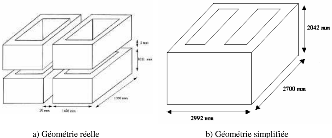
Figure IV-4. Représentation du circuit magnétique en vue de le modéliser
