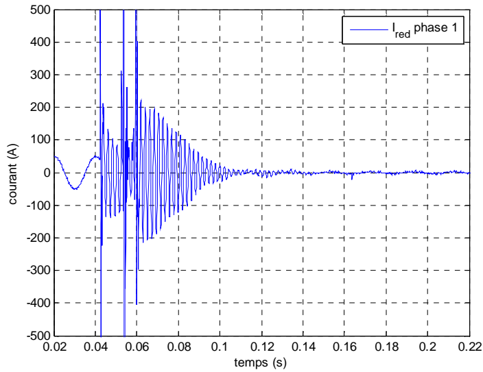
Figure II-17. Signal de courant après traitement (phase 1)
