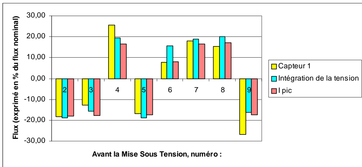
Figure V-37. Comparaison des méthodes pour l'estimation du flux rémanent
