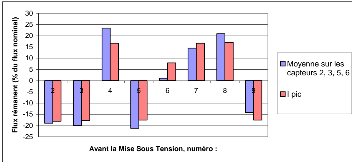
Figure V-35. Moyenne autour de l'estimation du flux sur les capteurs : 2, 3, 5, 6
