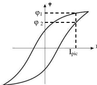
Figure III-8. Caractéristique d'une courbe « flux-courant »
