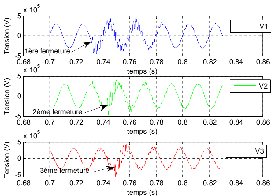
Figure II-4. Tensions simples mesurées en P2 lors de l'enclenchement de ligne
