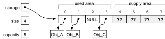
Figure 2: Manipulation d'un tableau avec trois variables: storage , size and capacity .
