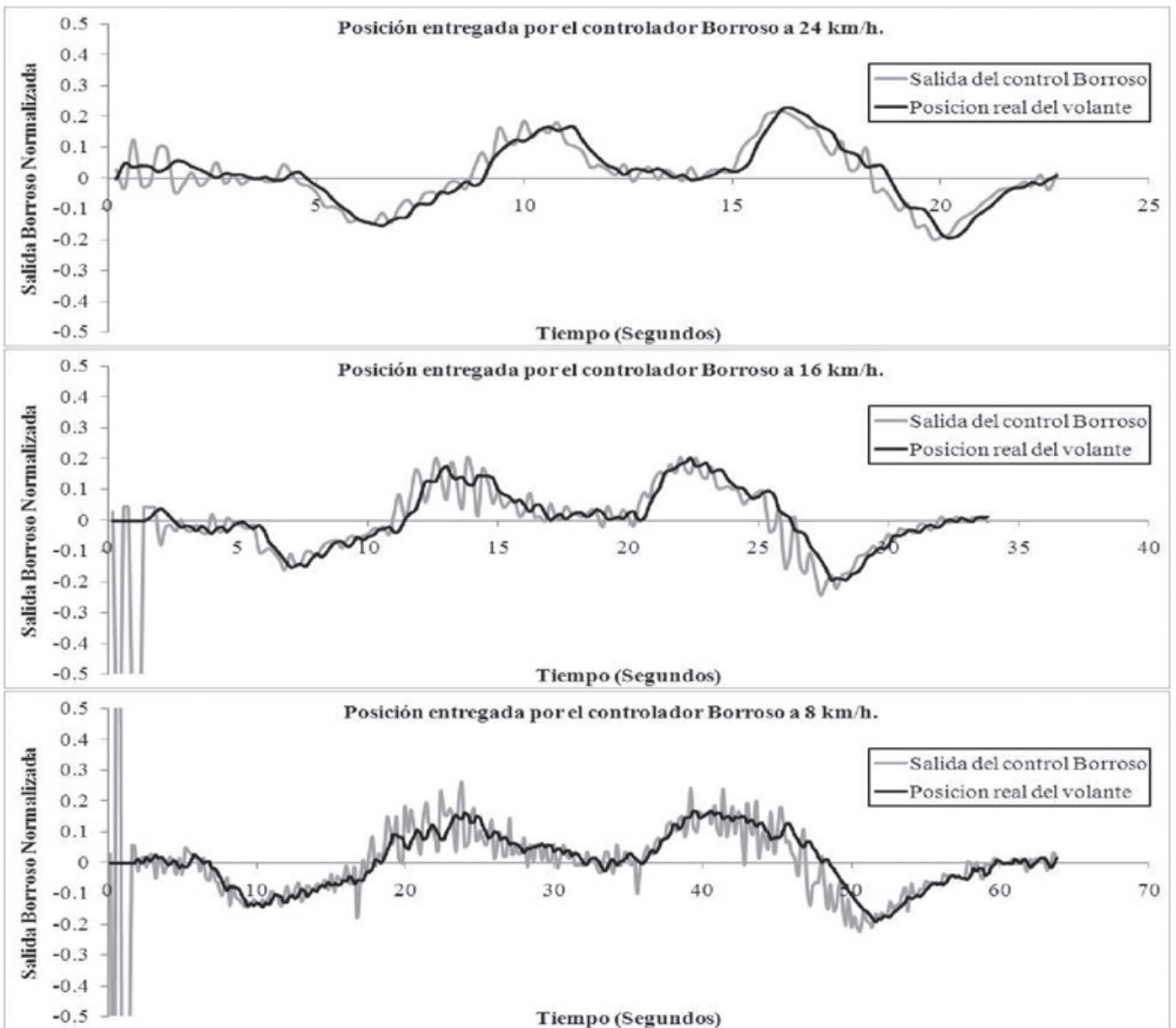
Fig. 8: Salida del controlador para la posición del volante en curvas poco pronunciadas
