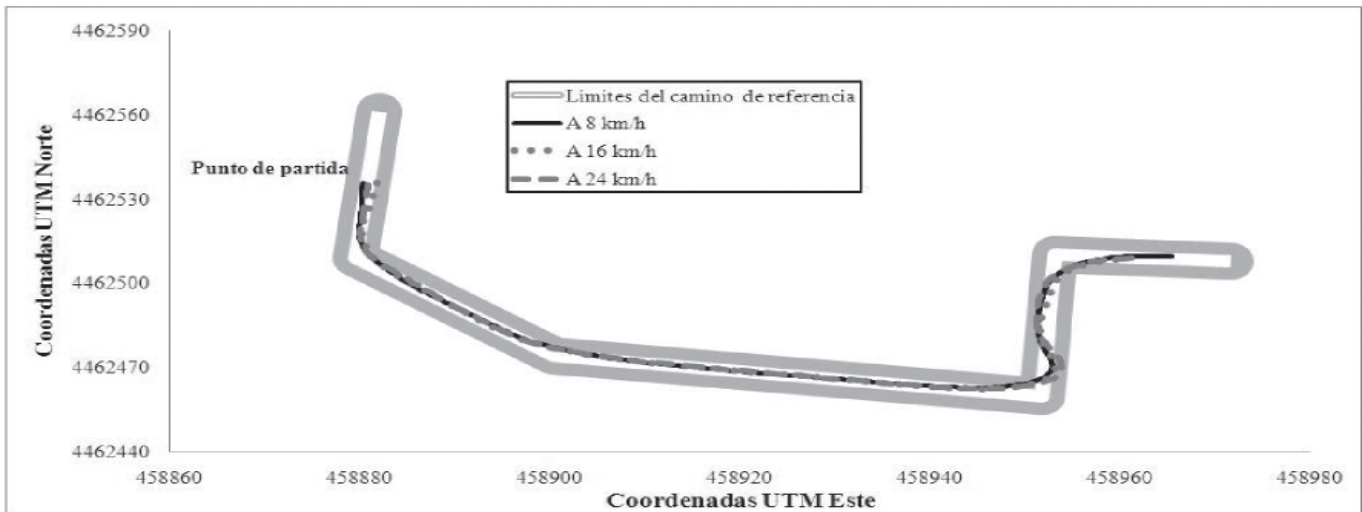
Fig. 9: Recorrido con curvas de mayor radio de curvatura
