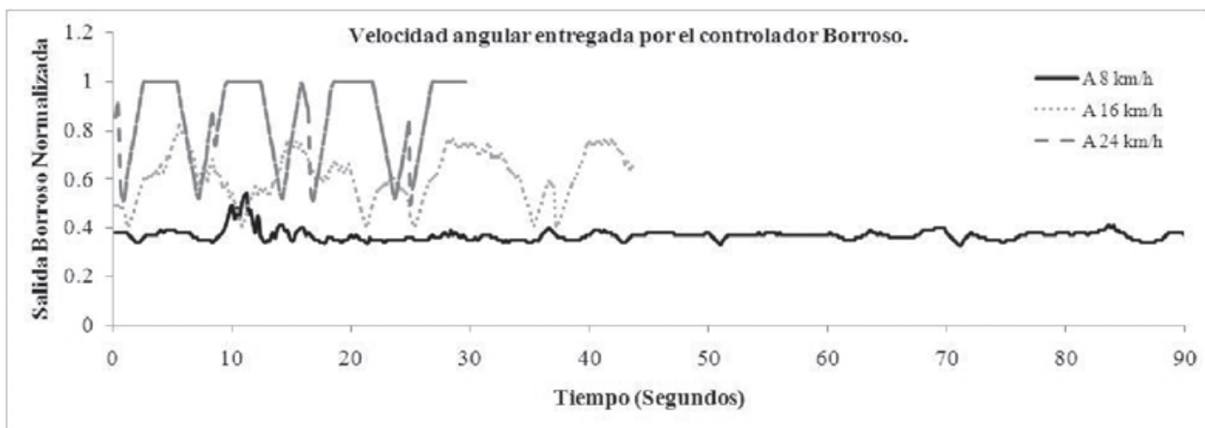
Fig. 10: Velocidad angular dada por el controlador en curvas más pronunciadas
