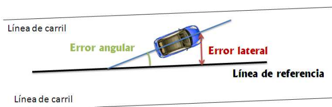
Fig. 4. Representación gráfica de las variables de entrada al controlador borroso.
