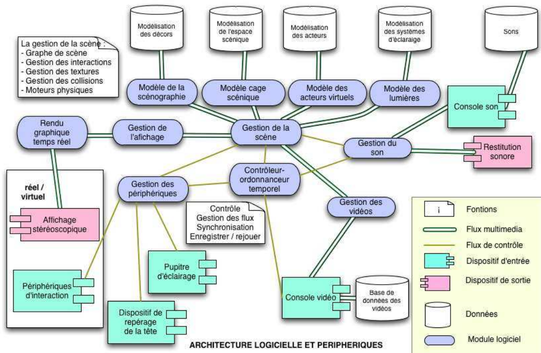
Figure 3 : Architecture logicielle et interactions dans THALIA
