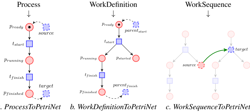
Figure 4. Transformations élémentaires composant SimplePDLToPetriNet
