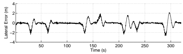
Fig. 7. Lateral error.
