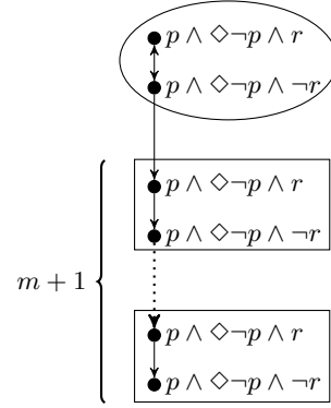
Fig. 15: META-REPL( p, n, m )
