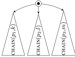
Fig. 3: s_{(k,l,m)}
