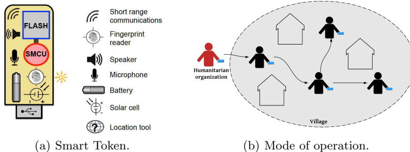
Fig. 1: Folk-IS paradigm.
