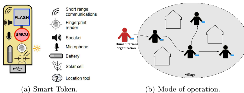
Fig. 1: Folk-IS paradigm.
