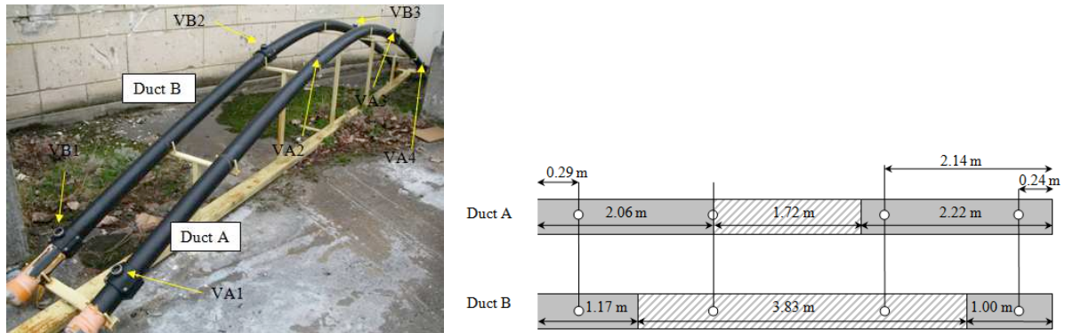
Figure 6 : Maquettes de conduits de précontrainte extérieure (laboratoire du CEREMA de Trappes) ; les zones hachurées représentent les vides et les ronds (o) les événements.
