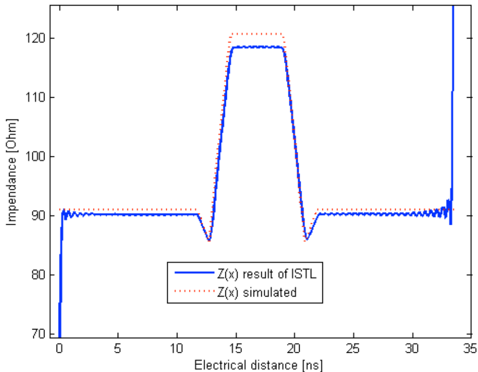
Figure 5 : Impédance simulée et inversée en fonction de la distance électrique x
