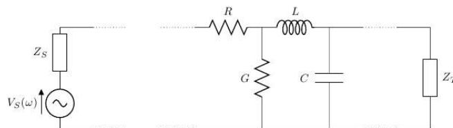
Figure 2 : Modèle de ligne de transmission intégrant la partie générateur (VNA) et l'impédance de charge
