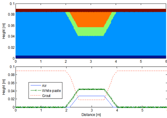
Figure 3 : Profil de remplissage du conduit de précontrainte extérieure simulé
