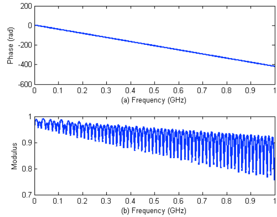
Figure 4 : Coefficient de réflexion S_{11} simulé
