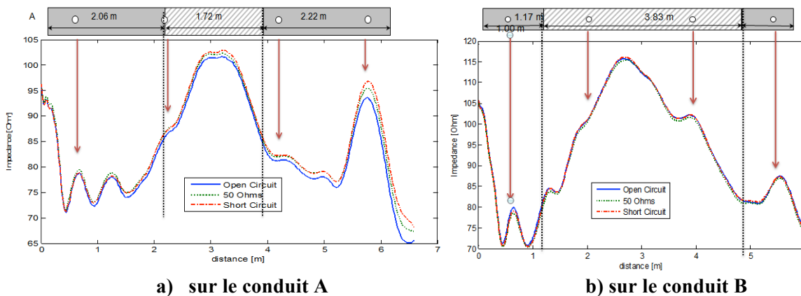
Figure 7: Le profil d'impédance calculée par rapport à marteler ISTL auscultation
