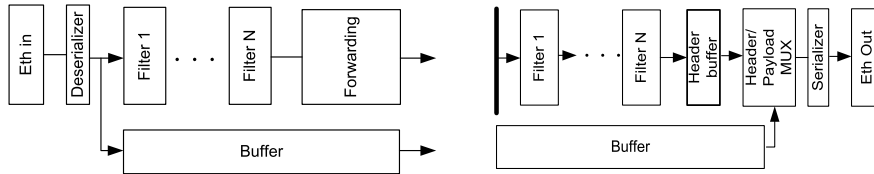
Fig. 2. Input port module
