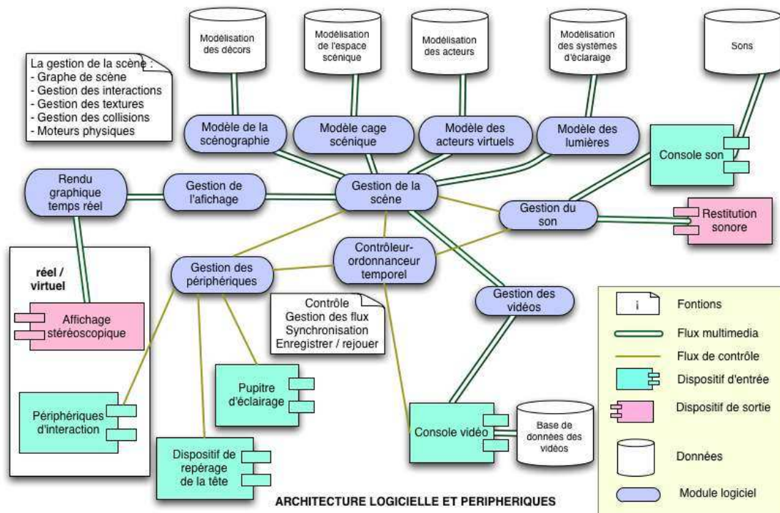
Figure 3 : Architecture logicielle et interactions dans THALIA
