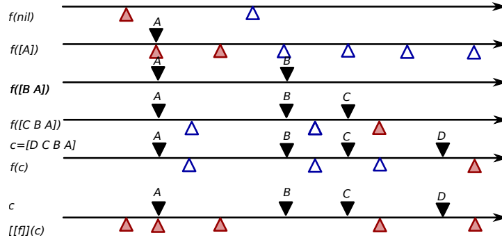
FIGURE 4 – Exemple de la fonction \llbracket f \rrbracket
