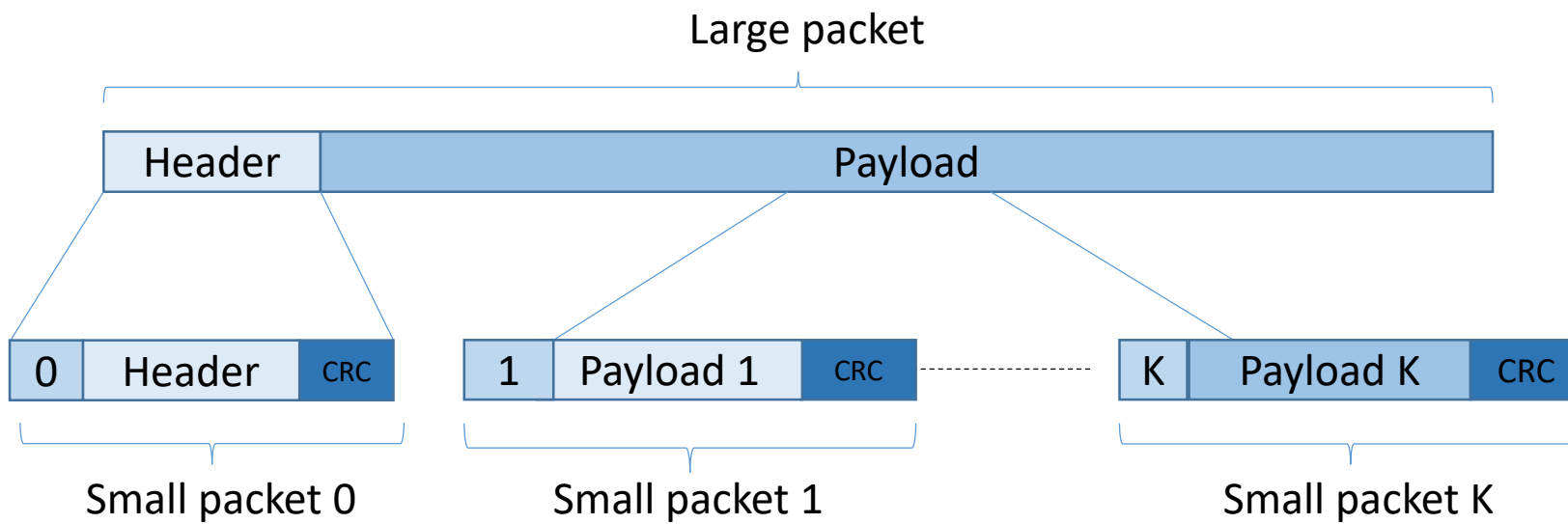
a) MAC Layer Frame
