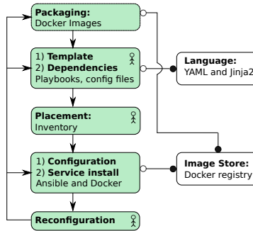
Fig. 2. Kolla model
