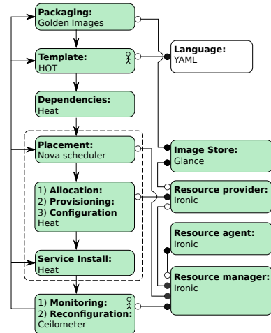
Fig. 6. TripleO model
