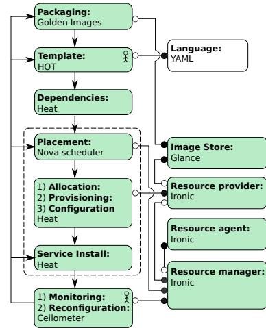
Fig. 6. TripleO model
