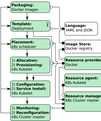
Fig. 5. Kubernetes model
