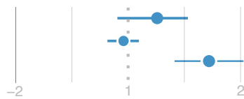
Figure 4: Exemple d'intervalles de confiance pour un quotient.
