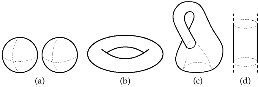
FIGURE 1.5 – Quelques exemples de surfaces topologiques. (a) Une surface non connexe (deux composantes connexes). (b) Une surface de genre non nul : le tore. (c) Une surface non orientable : la bouteille de Klein. (d) Une surface non bornée : le cylindre infini.
