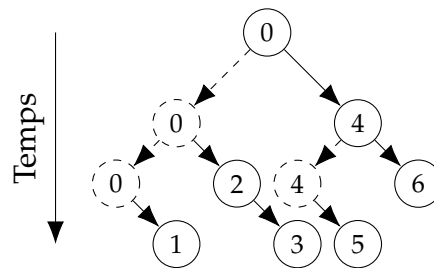
FIGURE 1 – Exemple d'arbre binomial avec 5 destinataires. Les étiquettes des sommets correspondent au rang des différents nœuds dans le communicateur global. Chaque niveau de l'arbre est une étape de l'algorithme.
