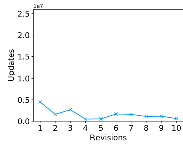
(i) Wikidata object updates
