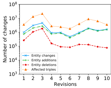
(g) Entity changes for Wikidata
