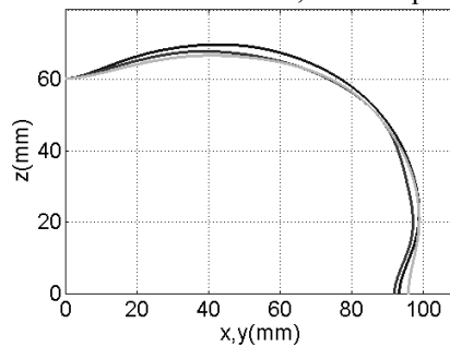
Figure 4 : Profils de la lentille n°B.4 dans les plans de coupe \varphi=0^\circ, 45^\circ, 90^\circ
