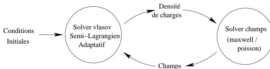
FIG. 1 – Boucle d'interaction
