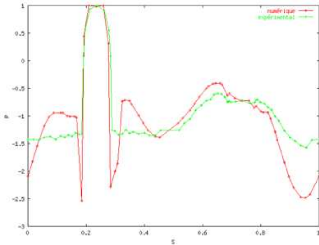
FIG. 11 – Profil de pression
