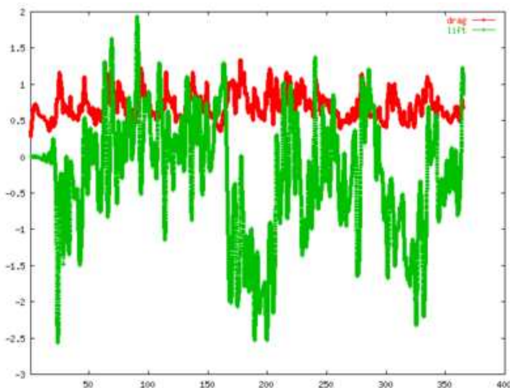
FIG. 41 – Évolution de la traînée et de la portance
