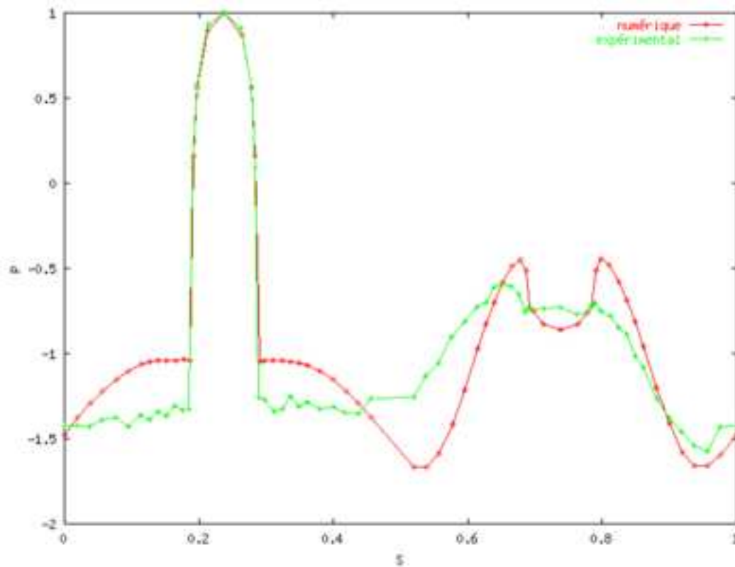
FIG. 29 – Profil de pression
