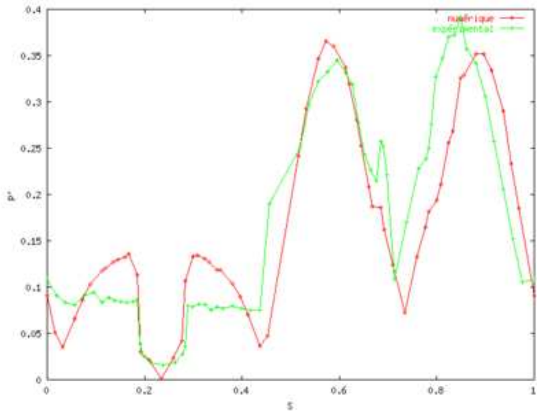
FIG. 8 – Profil de l'écart-type de pression
