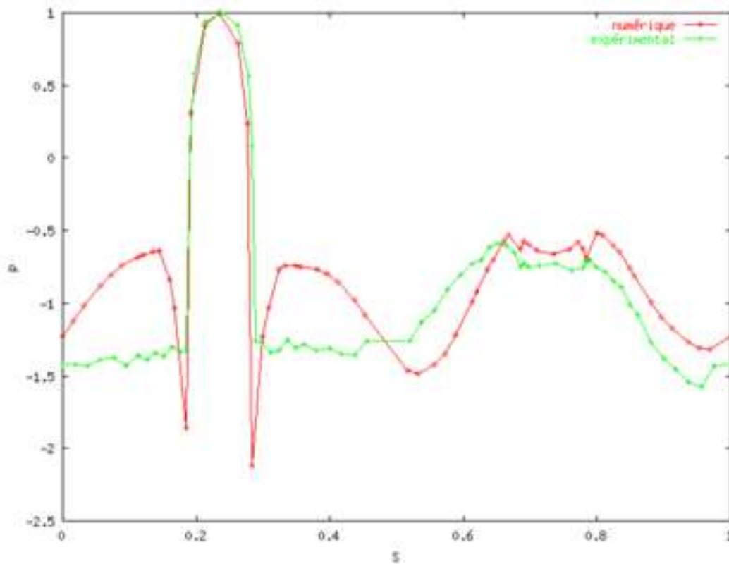
FIG. 17 – Profil de pression
