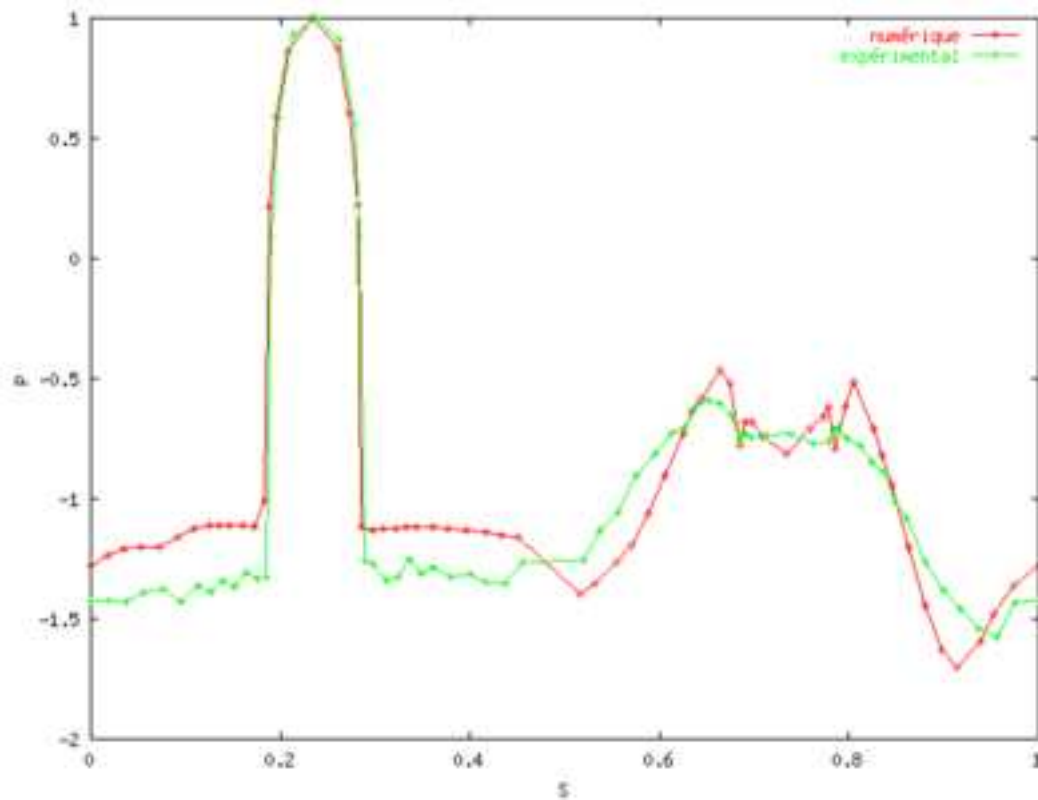
FIG. 39 – Profil de pression
