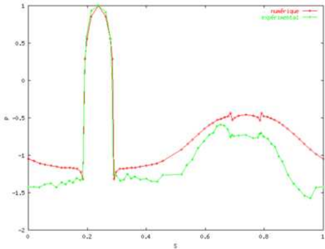
FIG. 26 – Profil de pression
