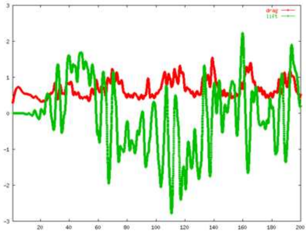
FIG. 38 – Évolution de la traînée et de la portance
