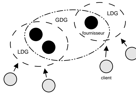
Figure 1: Architecture hiérarchique de JuxMem.
