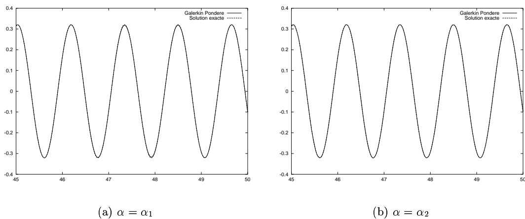
FIG. 13 – Composante E_z : évolution en temps / Raffinement 1:4 / Maillage : \lambda/16
