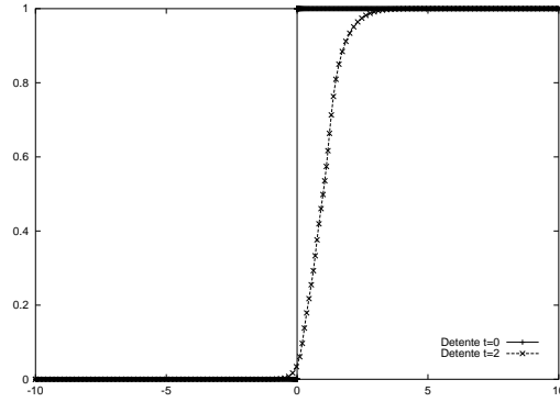
FIG. 41 – Déténtes à t = 0 (1000 nœuds) et t = 2 (138 nœuds).
