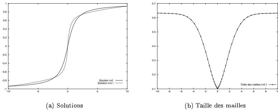
FIG. 4 – Solutions et taille des mailles à t = 0 et à t = 0.1 avec \alpha = 0.01 .
