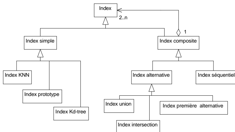
Figure 10 : diagramme de classes des index
