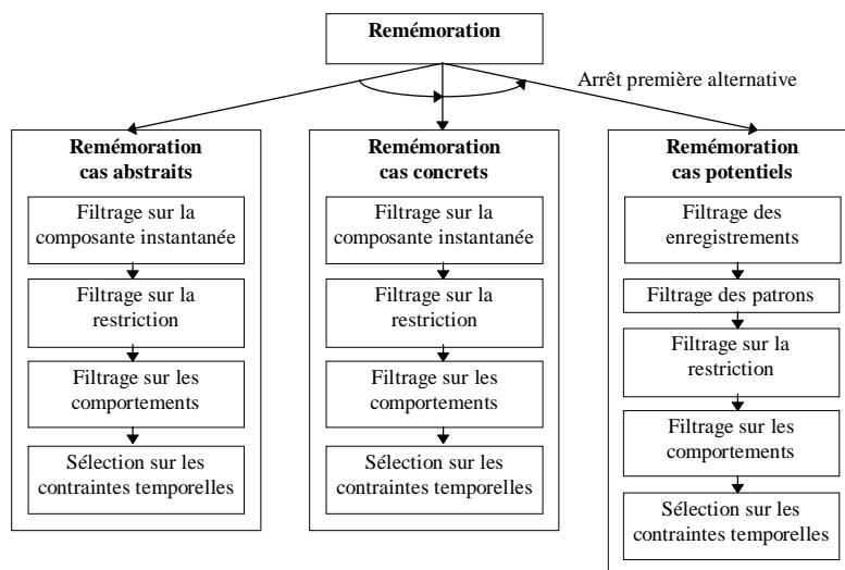
Figure 9 : décomposition en étapes de la stratégie de remémoration
