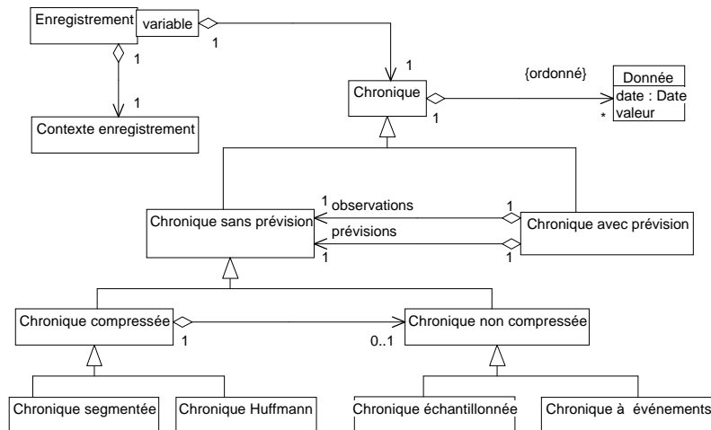
Figure 5 : diagramme de classes des enregistrements et des chroniques (notation UML, cf. annexe)
