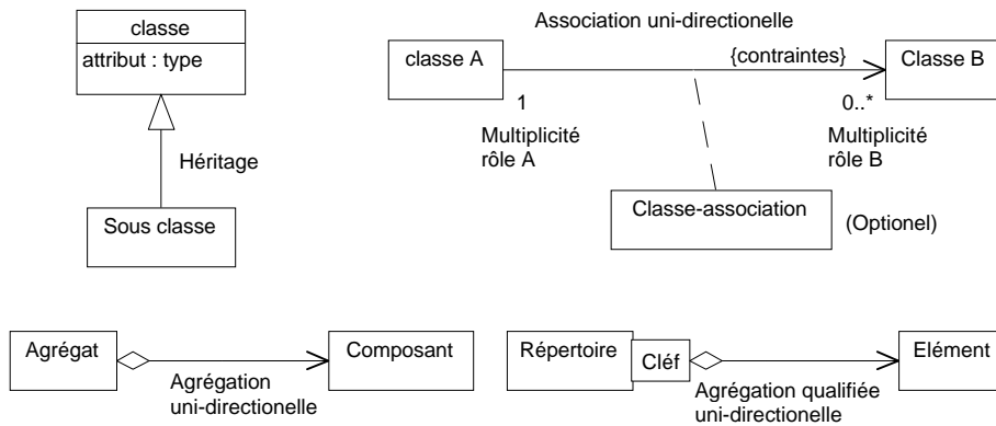
Figure 12 : éléments utilisés de la notation UML
