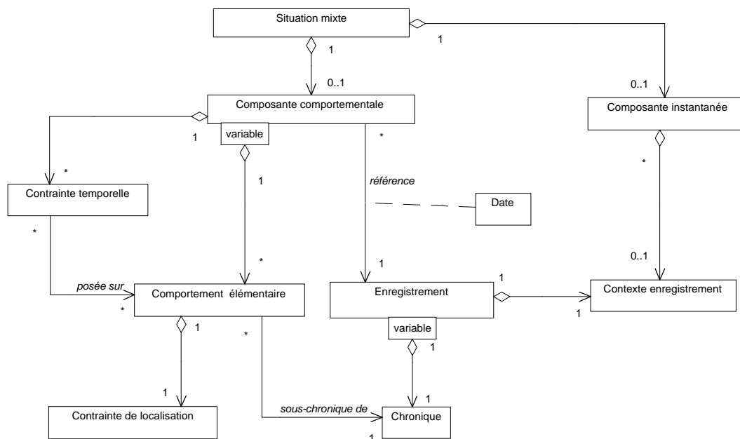
Figure 6 : diagramme des classes pour la représentation des situations comportementales
