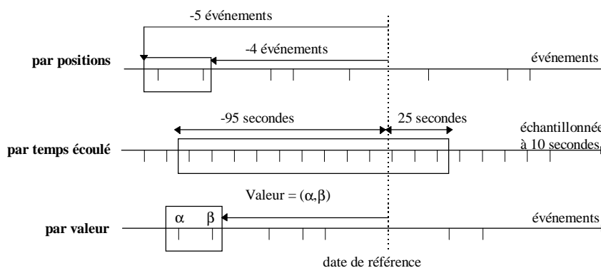
Figure 7 : exemples de contraintes de localisation
