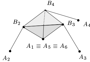
FIG. 10 – Manipulateur à trois articulations doubles sur la plate-forme et une articulation triple sur la base.
