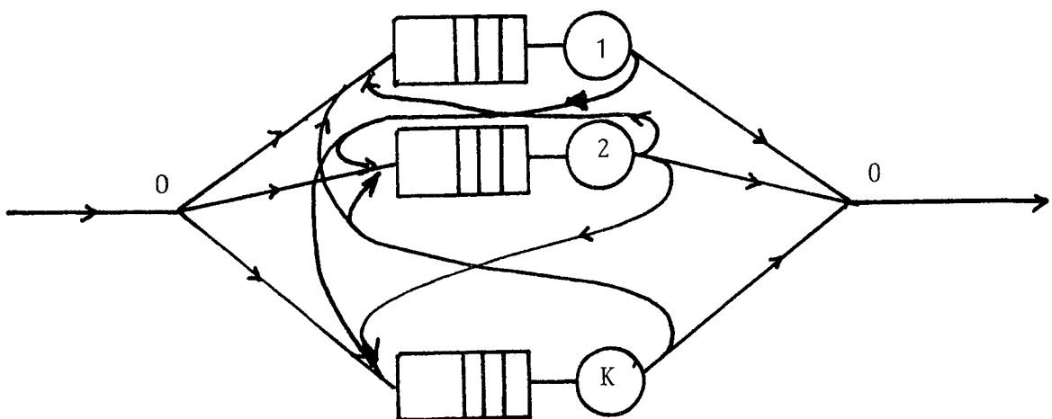
Figure 1: Un réseau général
