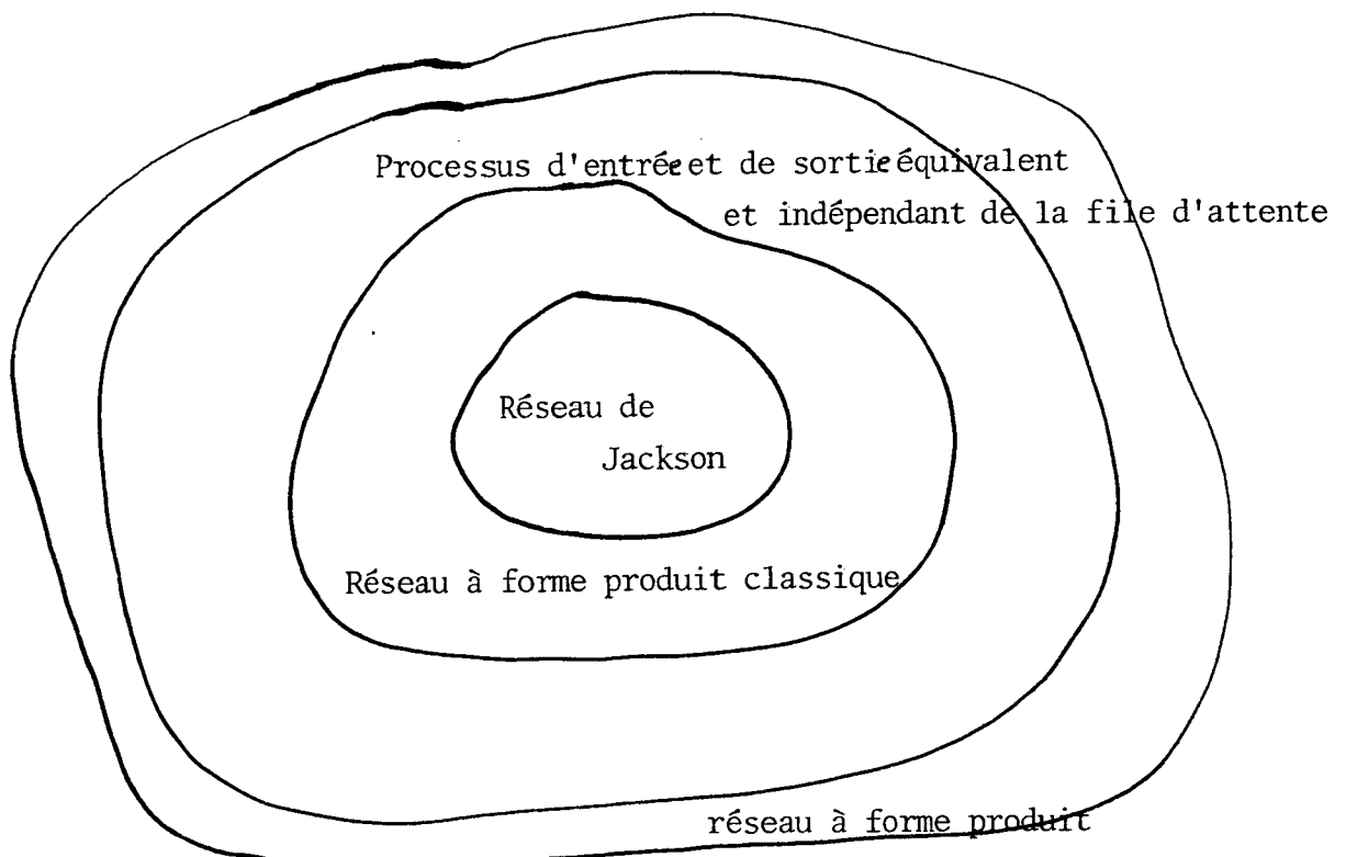
Figure 4: Réseau à forme produit
