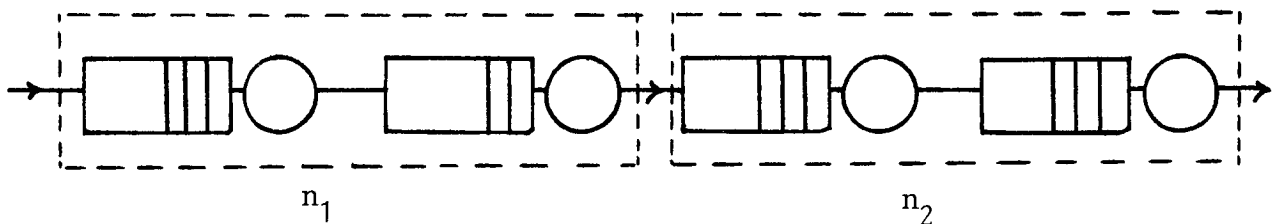
Figure 5: Réseau à forme produit non classique
