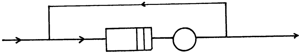
Figure 3: Une file d'attente M/M/1 avec rebouclage
