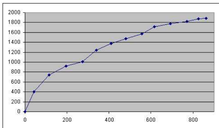
FIG. 3 – Evolution de la taille de la grammaire LTAG générée en fonction de la taille du corpus.
