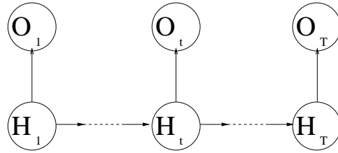
Figure 1: un HMM représenté comme un réseau Bayésien
