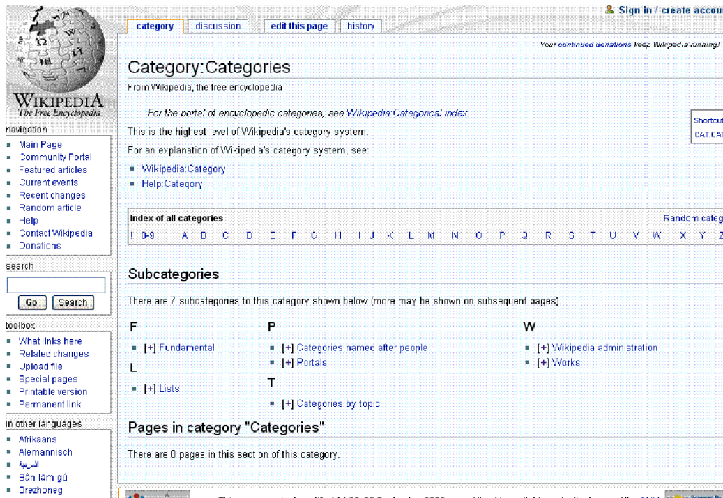
FIG. 1.3 – la catégorie des catégories.
