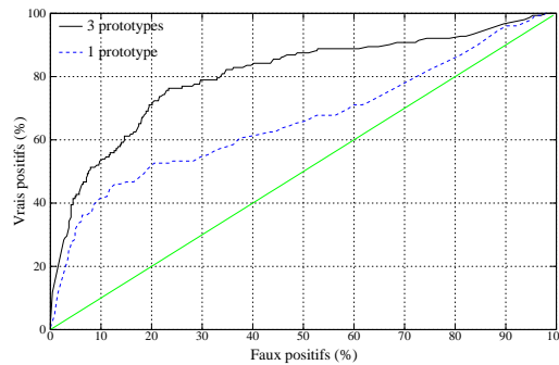
FIG. 4. Courbes ROC pour la reconnaissance des complexes K.
