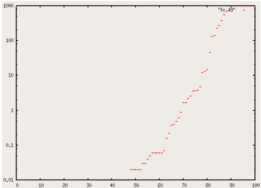
FIG. 2 – Répartition des temps du Forward-Checking pour 49% de trous.
