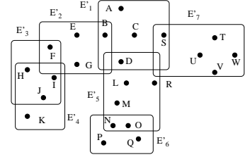
FIG. 2 – Dans ce recouvrement, ni la connexité ( E'_6 = E_{11} \cup E_{12} ), ni l'unicité ( E_5 \subset E'_4 \cap E'_3 ) et donc les séparateurs (e.g. E'_4 \cap E'_3 ) ne sont vérifiés. Ce recouvrement appartient en fait à \mathcal{CAH}_{G,H}[C^+] .
