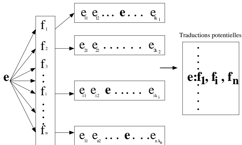
FIG. 4 – Identification des traductions potentielles d'un mot par symétrie
