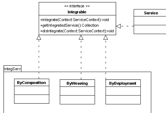
Figure 7. Diagramme de classe du service IntegServ
