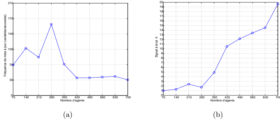
Fig. 5. Fréquence moyenne de mise à jour en termes d'attributs par seconde mesurés sur le gestionnaire sous différent nombre d'agents (a). Fonction rapport signal bruit d'une activité de supervision sous différents nombre d'agents (b).
