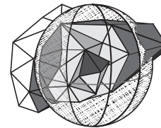
Figure 3: La RLI est composée de tous les tétraèdres contenus dans la sphère. Tous les tétraèdres colorés sont internes. Les gris clairs sont complets, les foncés sont de bord. Le tétraèdre central est le tétraèdre racine.
