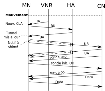
Figure 3. Séquence de messages lors d'un mouvement
