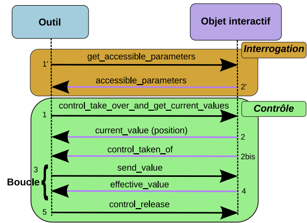
FIG. 1: Séquence de dialogue entre un outil et un objet interactif.
