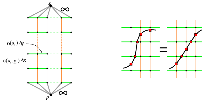
Figure 2. À gauche : graphe correspondant à l'énergie (8). À droite : si le coût et la pénalité sont uniformes, il y a ambiguïté. Les deux coupures ont exactement la même valeur : trois arcs de coût (les carrés) et 2 arcs de pénalité (les ronds)
