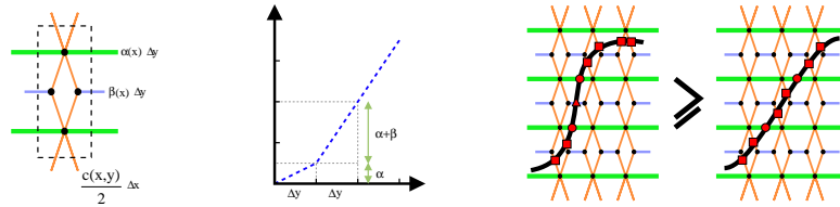
Figure 3. À gauche : l'élément de base utilisé. Au milieu : la fonction de pénalité p_{conv} correspondante. À droite : une variation continue est moins pénalisée qu'un palier : elle coupe une pénalité secondaire de moins (triangle)
