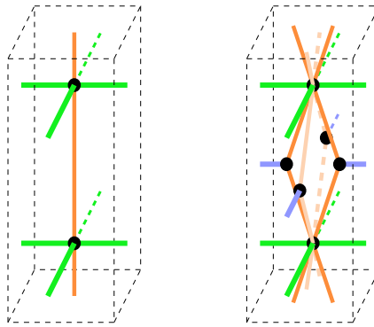
Figure 4. Gauche : l'élément de base utilisé pour une pénalité linéaire. Droite : pour une pénalité convexe
