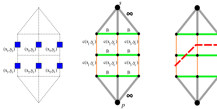
Figure 1. Un exemple simple. À gauche, les positions possibles pour f et la structure du graphe en pointillés (les positions sont associées à des arcs verticaux). Au milieu, le graphe avec les capacités des arcs. À droite, un exemple de coupure
