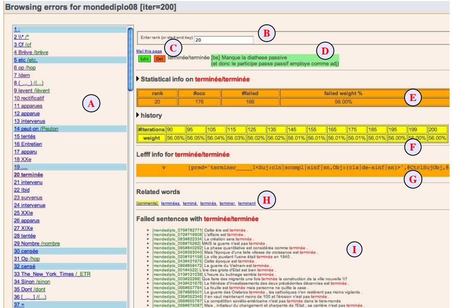
Figure 1. Visualisation du résultat de la fouille d'erreurs (illustré pour MD08/FRMG)
