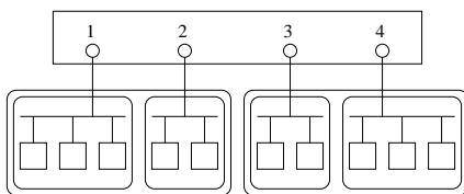
(b) avec VLAN : plusieurs domaines de collision, plusieurs domaines de diffusion
