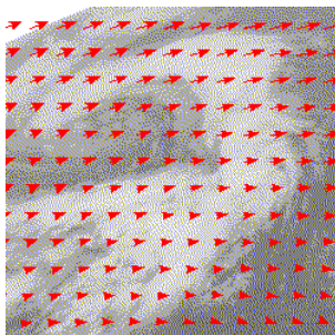
FIG. 2 — Vortex nuageux
