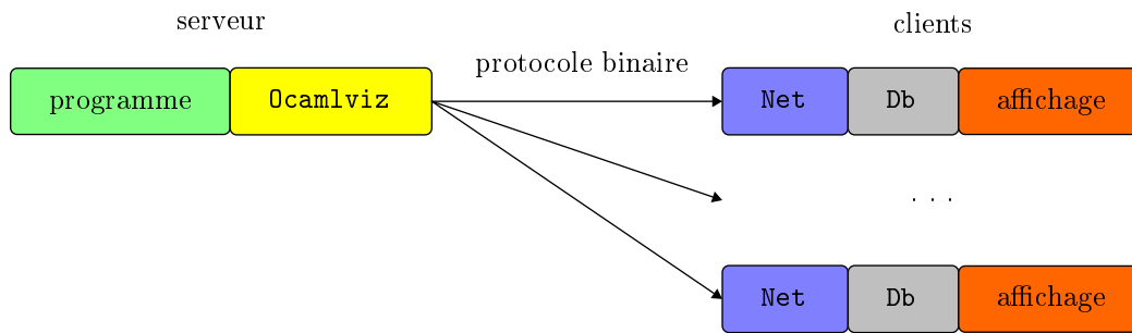
FIG. 6 – Ocamlviz est composé d’une bibliothèque liée au programme instrumenté, qui communique via le réseau avec un ou plusieurs clients.
