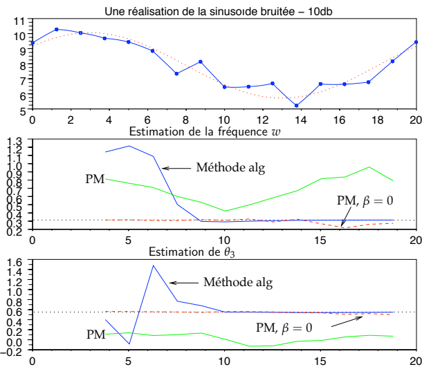
FIG. 2: Comparaison avec Prony modifiée : bruit coloré
