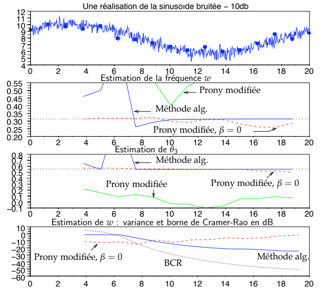
FIG. 1: Comparaison avec Prony modifiée l'estimation fournie par la méthode présentée est non biaisée et insensible à la perturbation \beta contrairement à la méthode de Prony modifiée (PM). C'est seulement en l'absence de la perturbation constante ( \beta = 0 ) que PM
