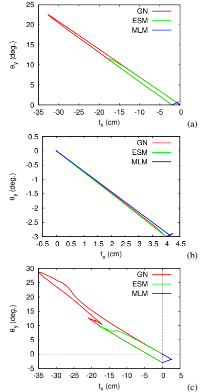
FIG. 2 – Chemin dans le sous-espace (t_x, \theta_y) des approches GN, ESM et MLM pour différentes tâches de positionnement. (a) tâche 1 ; (b) tâche 2 ; (c) tâche 3.
