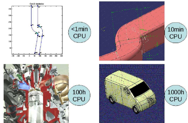
Fig. 7. Test Cases
